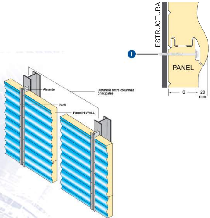
Detalle de la junta Longitudinal
